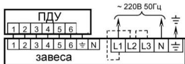
Схема подключения X409E10 к однофазной сети и пульту
