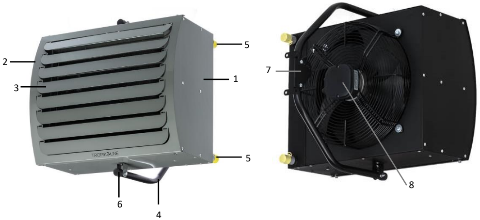
Рис.1. Устройство прибора
