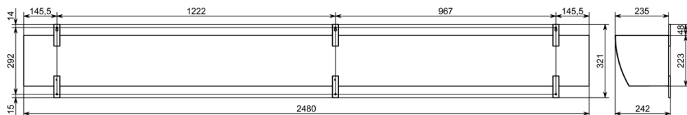
Рис. 2. Габаритные и установочные размеры приборов
