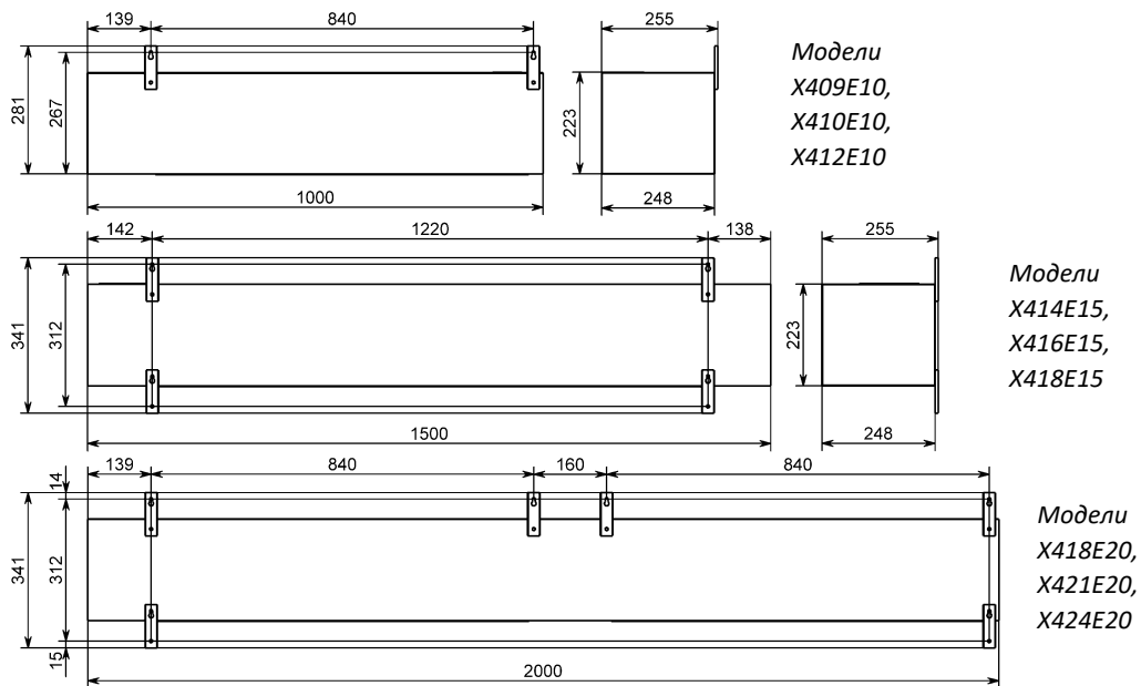
Рис. 2. Габаритные и установочные размеры приборов
