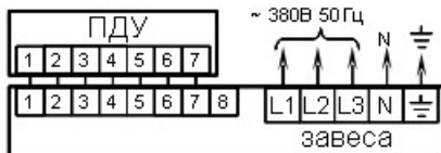
Рис. 3. Схема подключения занавес к электросети и пульту управления
