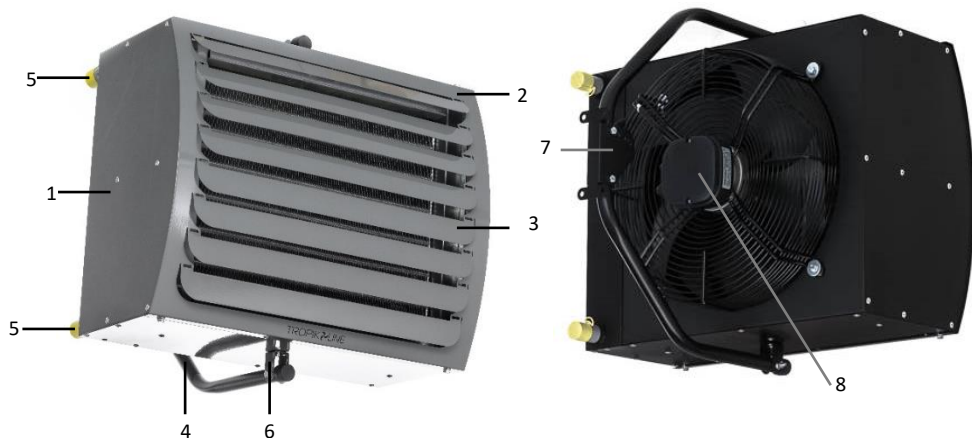
Рис.1. Устройство прибора
