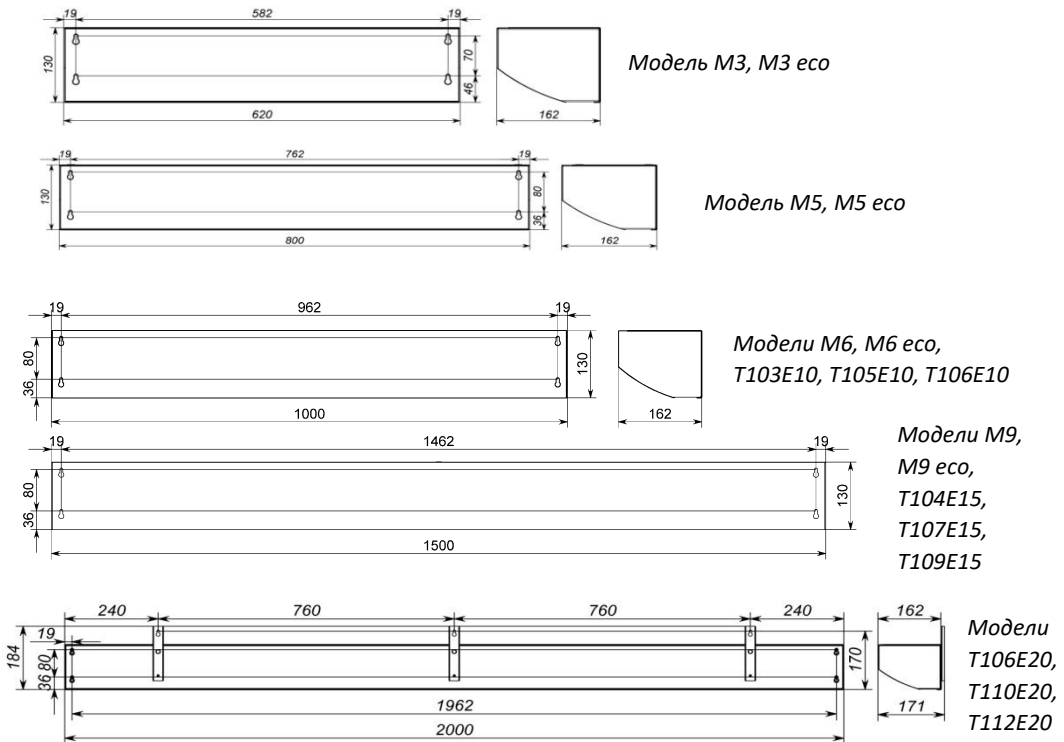
Рис. 2. Габаритные и установочные размеры приборов ( Установка кронштейнов - опционально )
